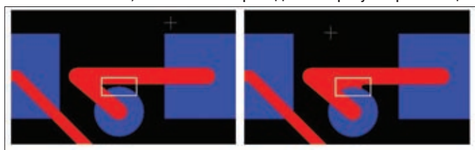
Рис.3. Диагностика и автоматическое устранение мест возможных подтравов
