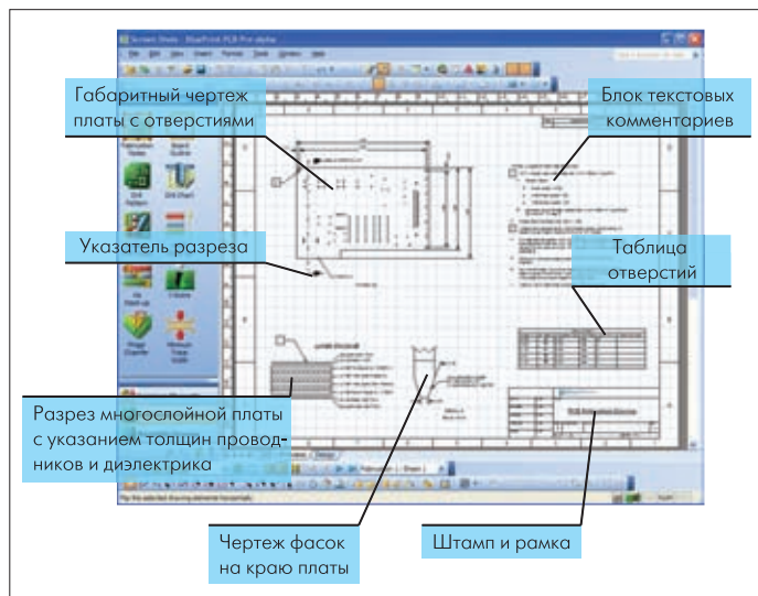
Рис.10. Отображение деталей процесса изготовления
