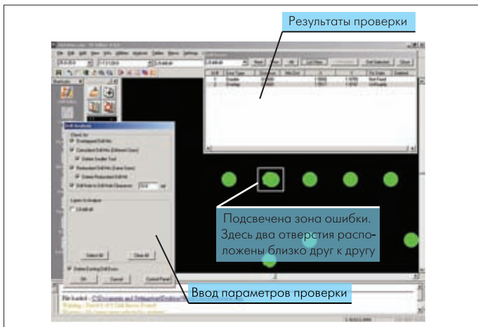
Рис.5. NC Editor – пример обнаружения ошибок сверления
